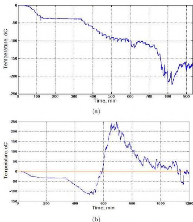
Рис. 2. Ход разностной температурной кривой в случае отсутствия реакции Ni+LiAlH 4 (а) и в случае ее наличия (б).
