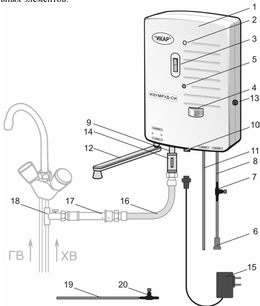
Рис. 1. Установка "Изумруд-СИ" (мод. 03): 1 – корпус; 2 – индикатор работы установки в режиме активации воды; 3 – выключатель режима получения анолита и католита; 4 – индикатор тока при работе в режиме получения активированных растворов; 5 – индикатор работы установки в режиме получения активированных растворов; 6 – фильтр раствора; 7 – вентиль регулировки подсоса минеральных добавок и раствора NaCl; 8 – шланг подсоса минеральных добавок и раствора NaCl; 9 – штуцер для подвода водопроводной воды к установке; 10 – разъем для подключения блока питания; 11 – шланг выхода анолита; 12 – излив для выхода очищенной питьевой воды и католита; 13 – гнездо предохранителя 10 А (может отсутствовать в установках с самовосстанавливающимся предохранителем); 14 – регулировочный кран; 15 – блок питания (с предохранителем на 2 А); 16 – шланг (длинный); 17 – фильтр МФГ; 18 – кран; 19 – трубка удлинитель; 20 – регулировочный кран потоков.
