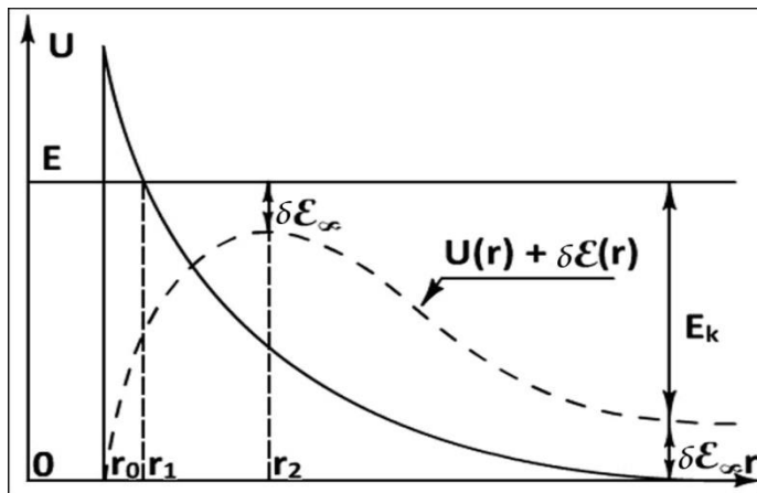
Рисунок 1. Схематическое изображение туннелирования заряженной частицы из ядра
